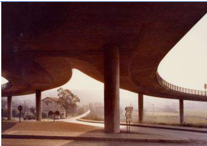
La Avanzada overpass. La Coruña. Spain (1972)
